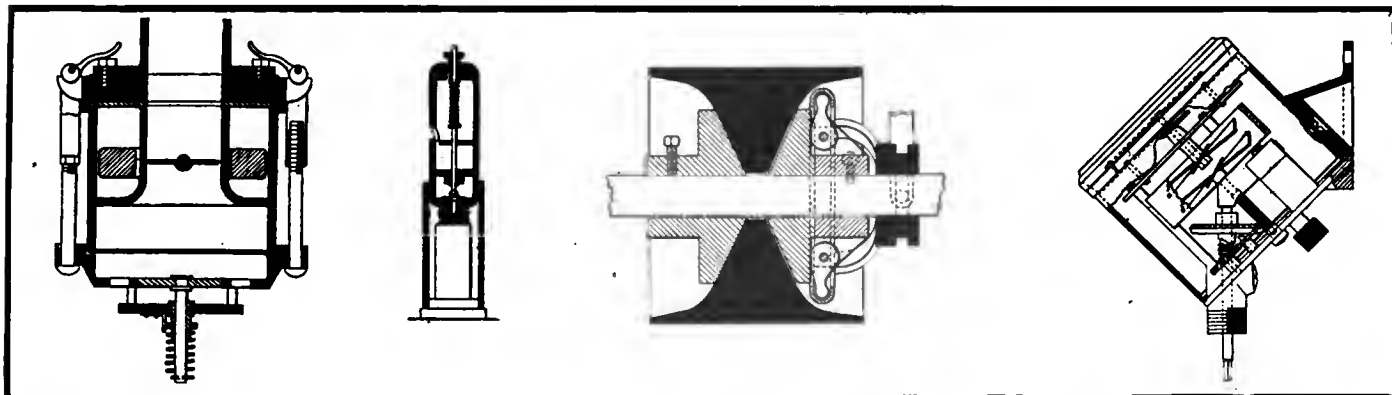
Fig. 1—Zisch carbureter
